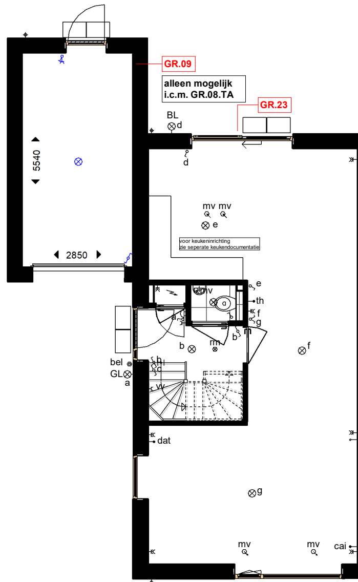
begane grond
