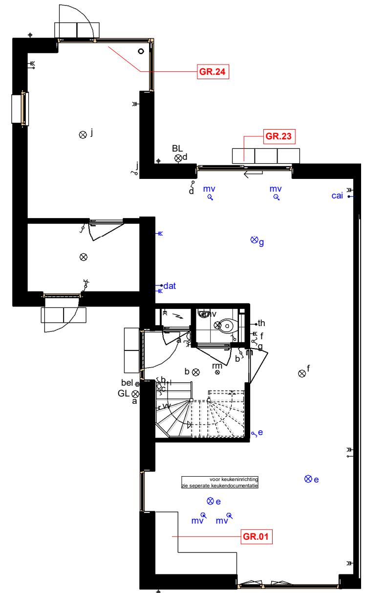
begane grond
