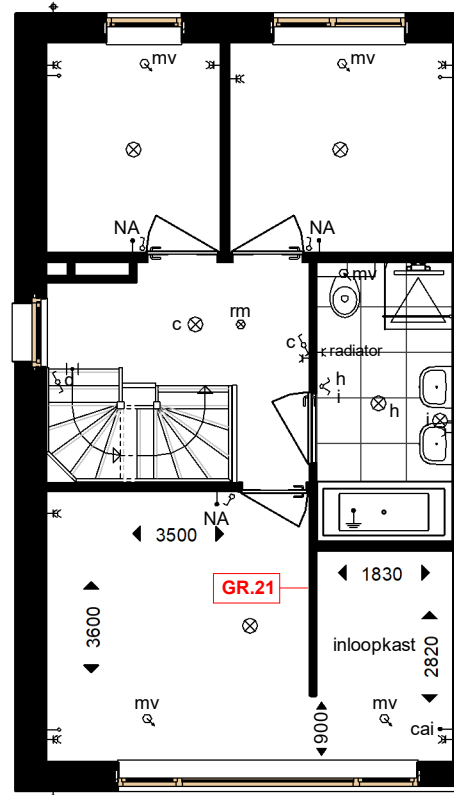
eerste verdieping
