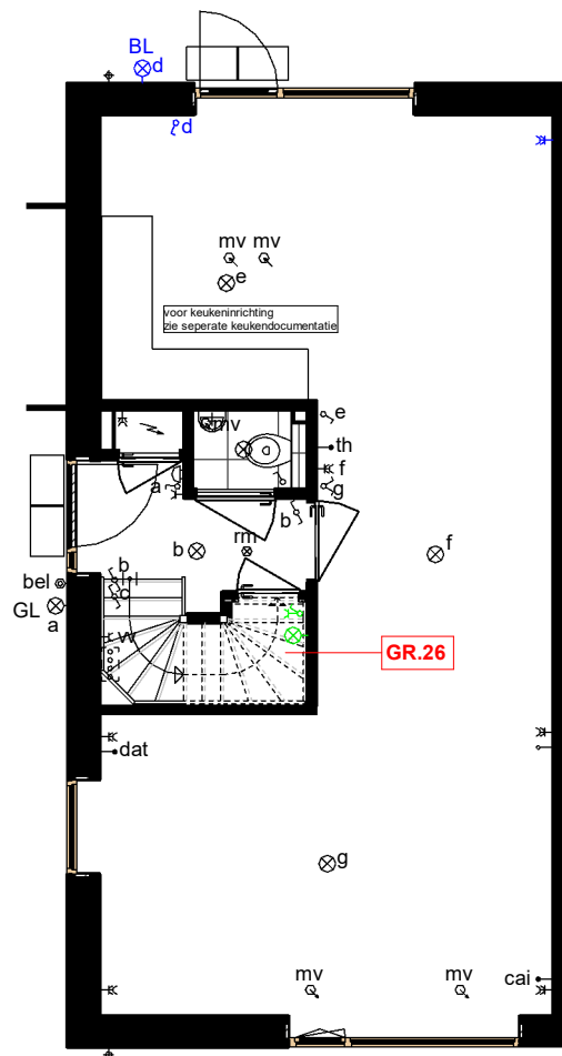
begane grond
