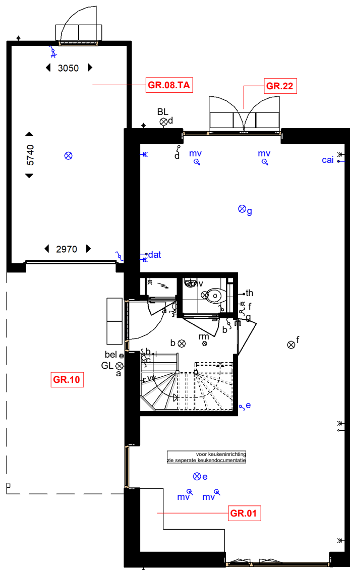
begane grond
