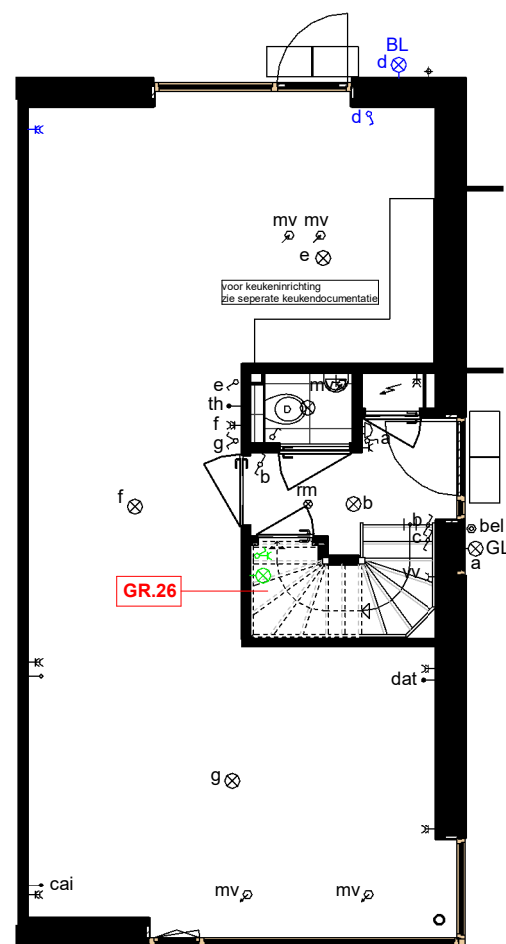
begane grond
