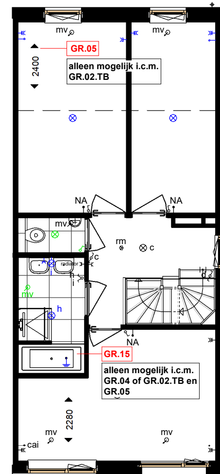
eerste verdieping
