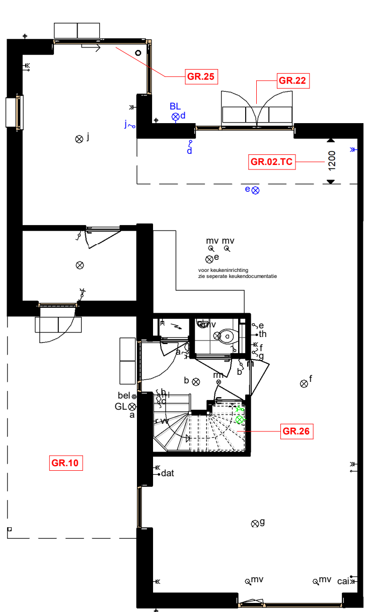
begane grond
