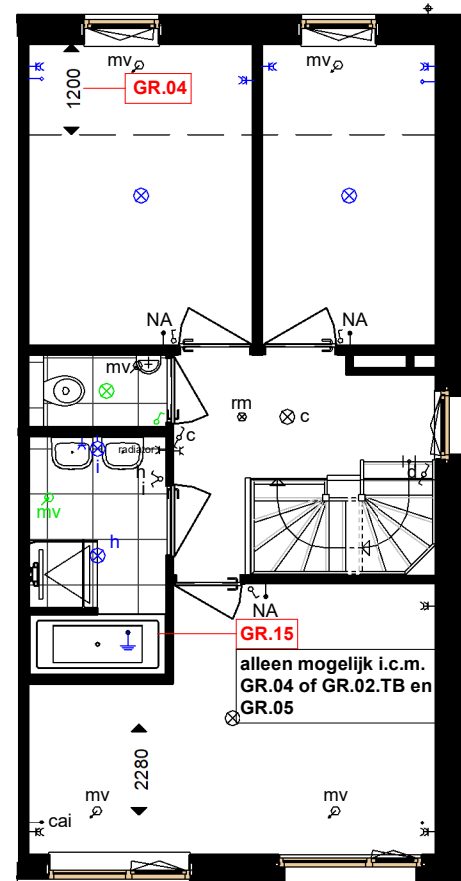
eerste verdieping
