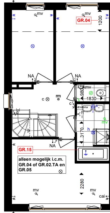
eerste verdieping
