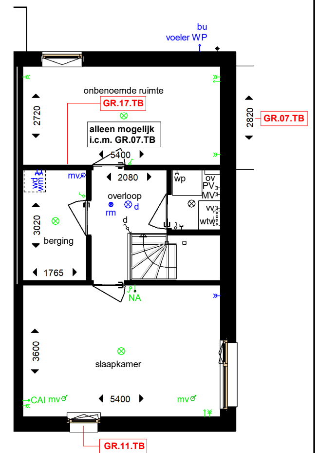
tweede verdieping
