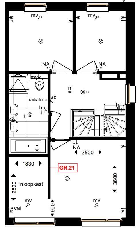
eerste verdieping
