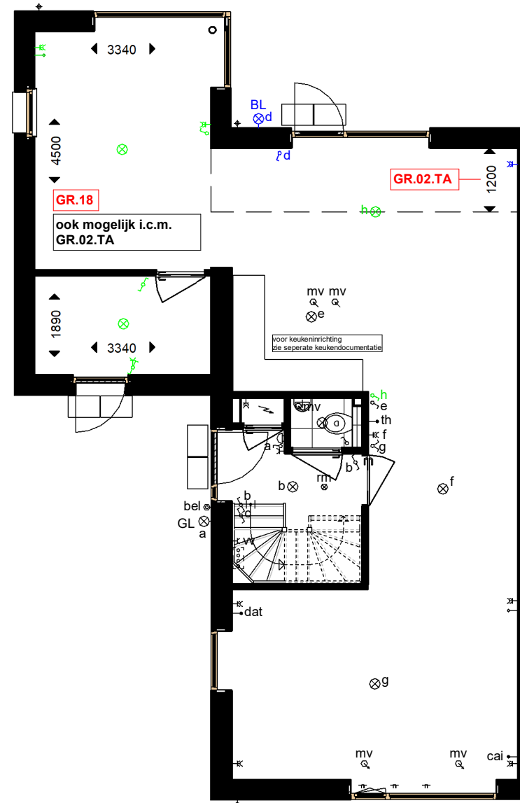
begane grond
