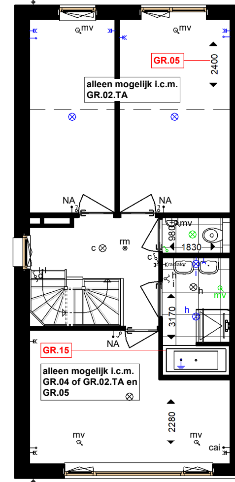
eerste verdieping
