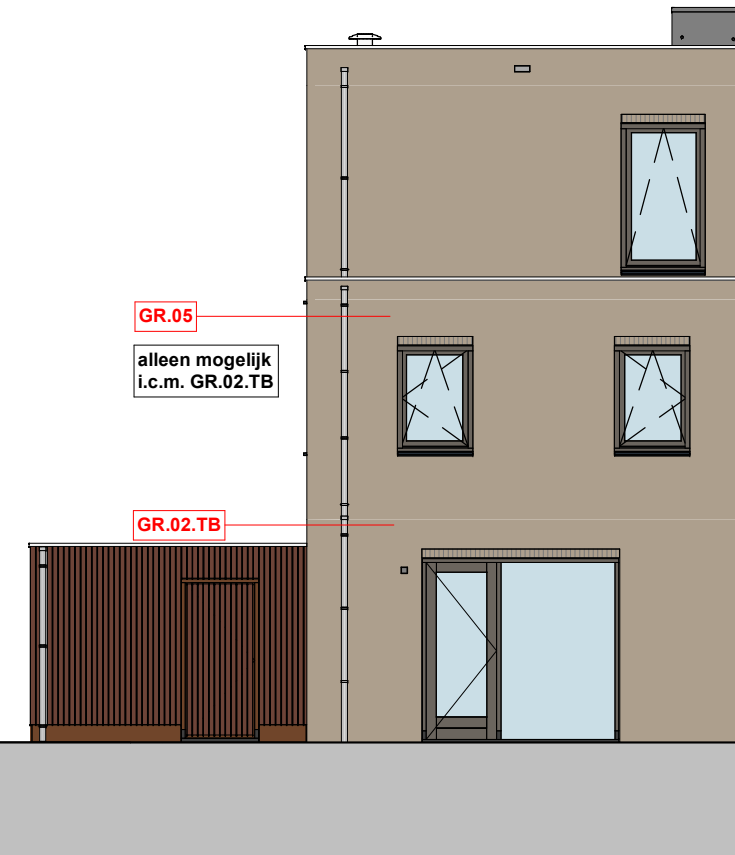
achtergevel
