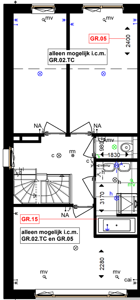
eerste verdieping
