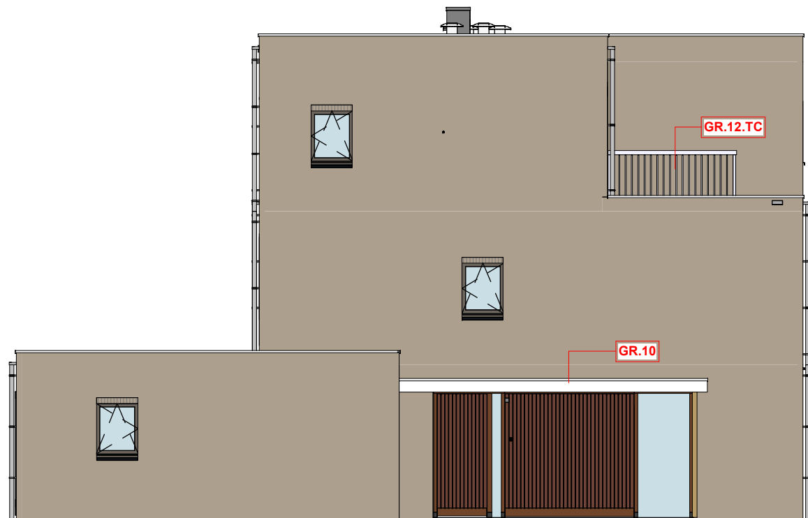
zijgevel
