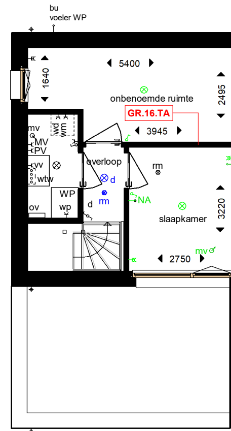
tweede verdieping
