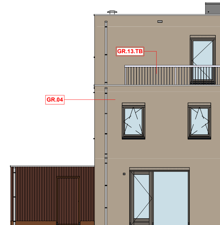
achtergevel
